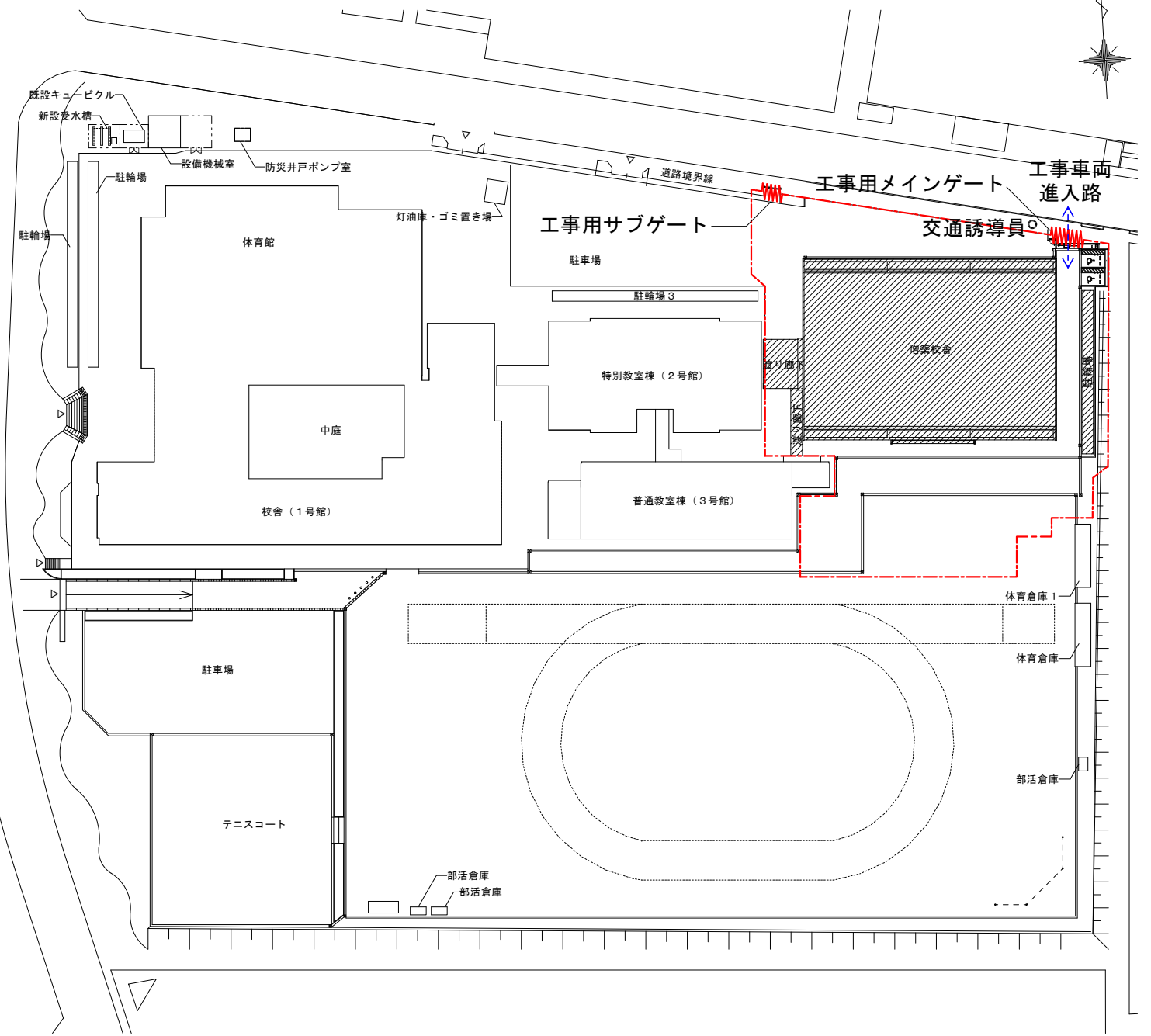
配置図
