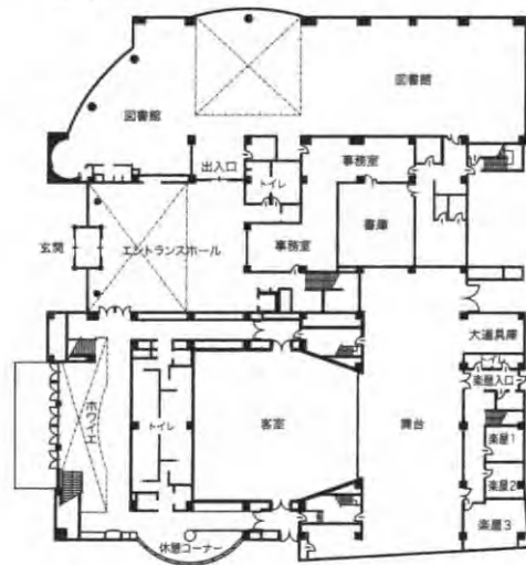
1階平面図
