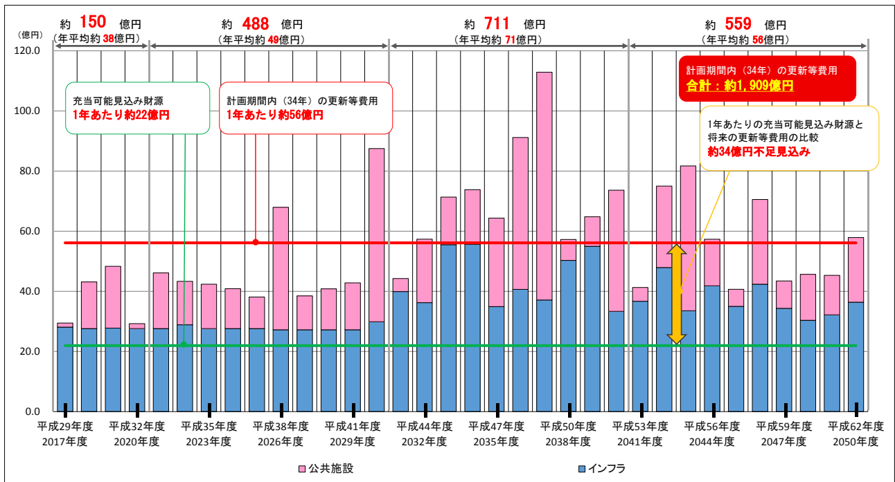
図 2-18 公共施設等の将来の更新等費用の推計
