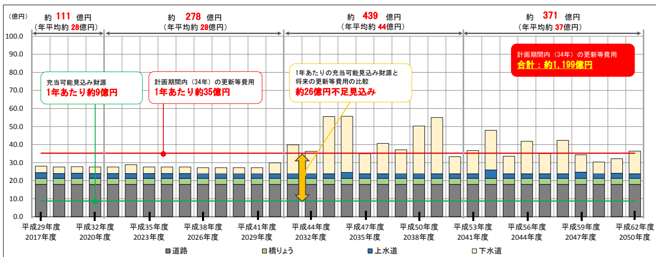
図 2-20 インフラ資産の将来の更新費用の推計
