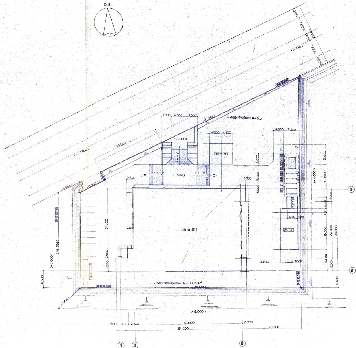
配座図 1:300
