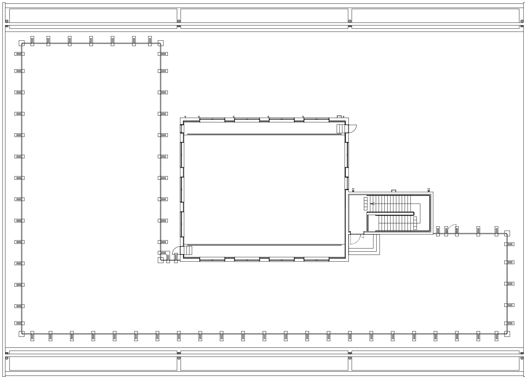
屋上平面図
