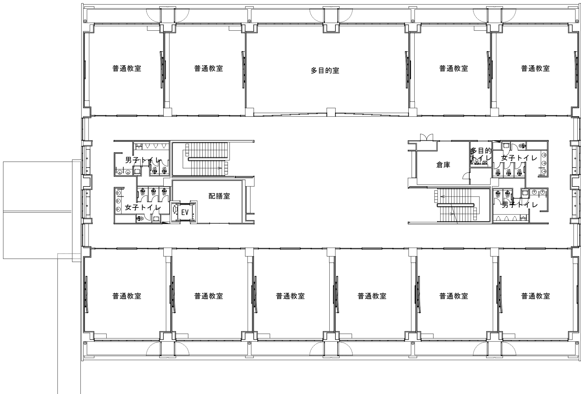
2 階 平 面 図
