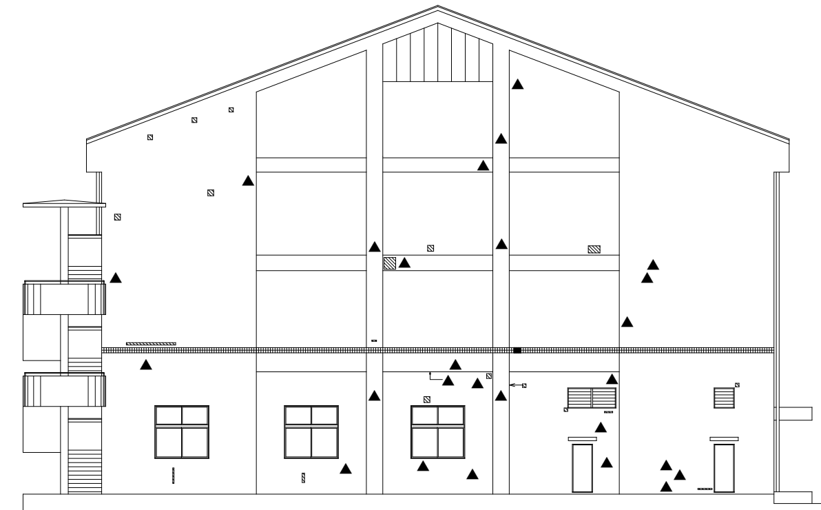
西側立面図
