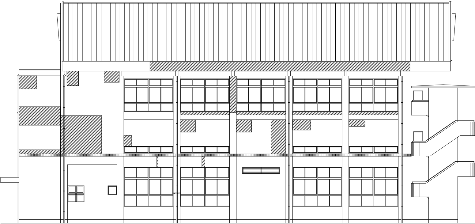
北側立面図
