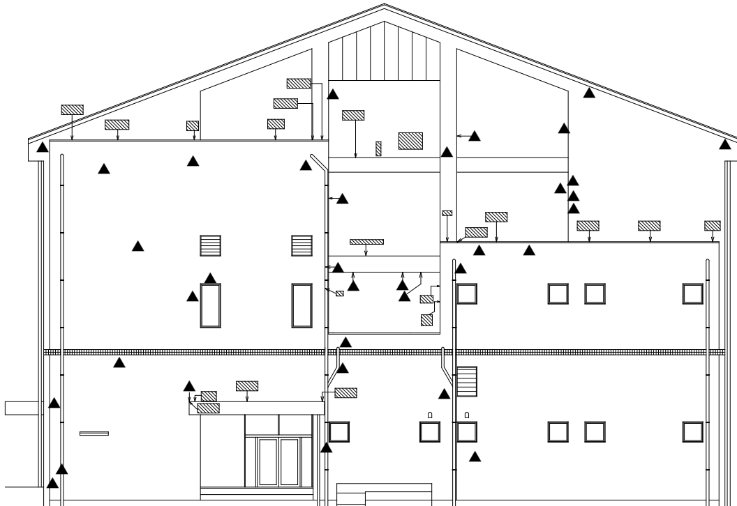
東側立面図
