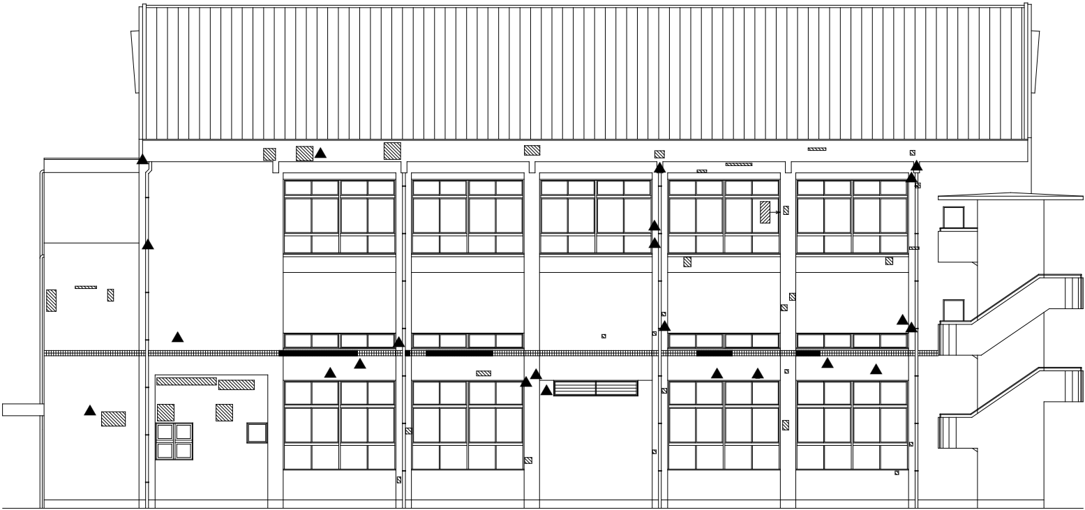
北側立面図
