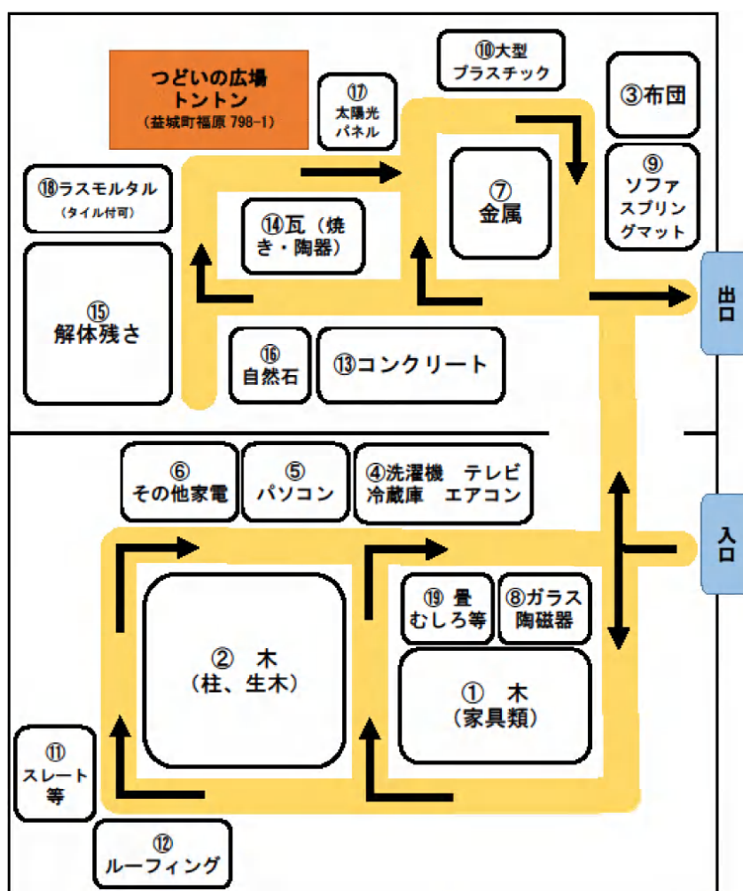
図 3-5 仮置場のレイアウト (地震災害発生時の設置例)
