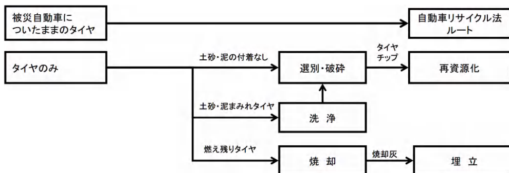
図 3-15 タイヤ類の処理フロー
