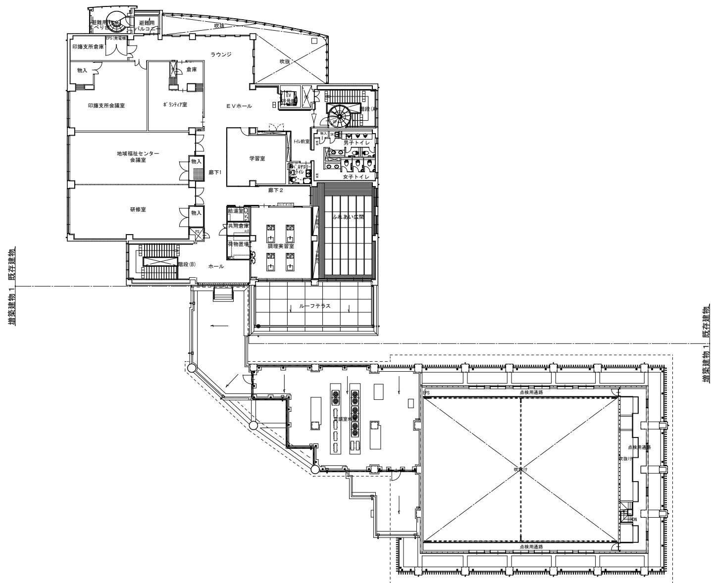
3階平面図（改修）
