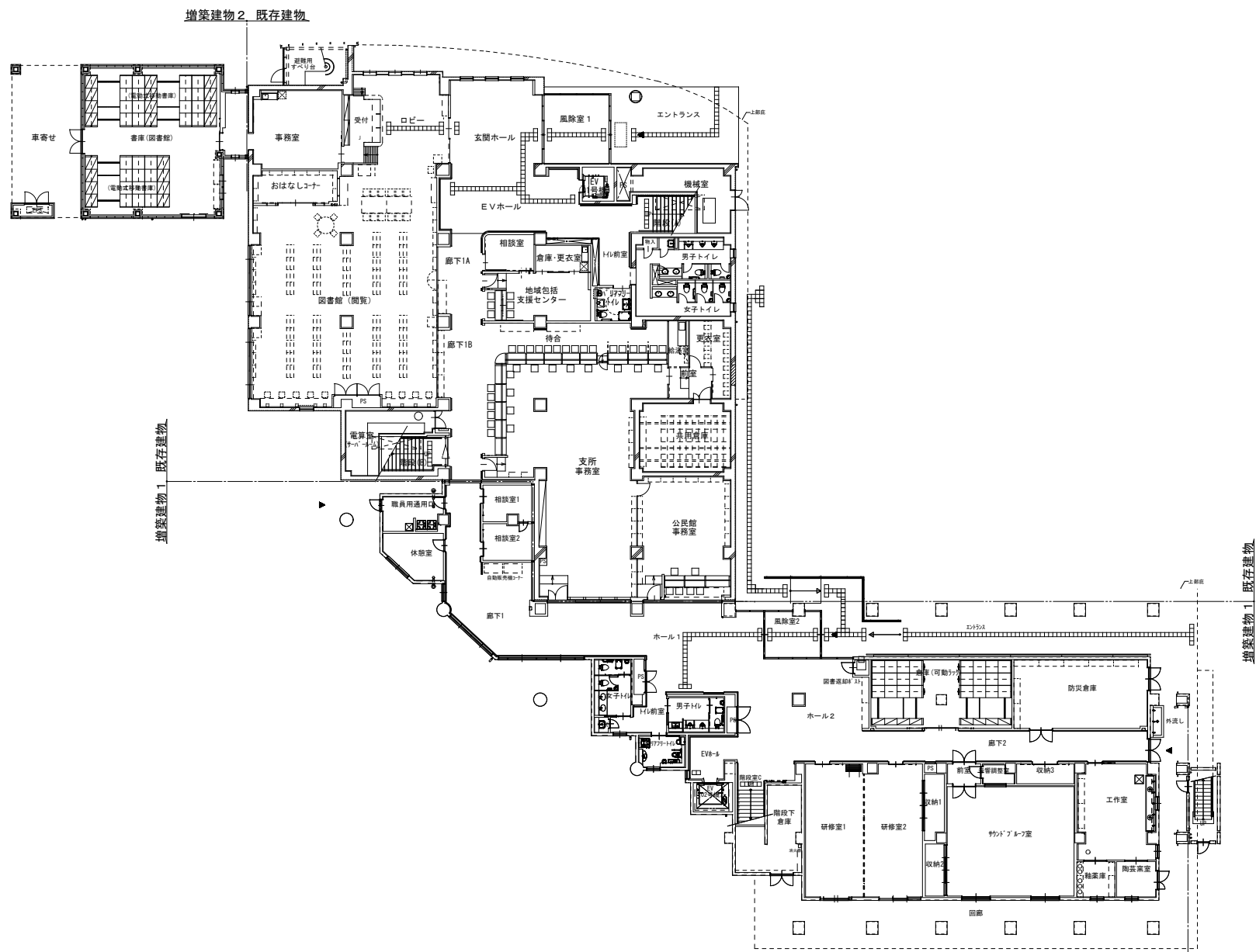
1階平面図(改修)
