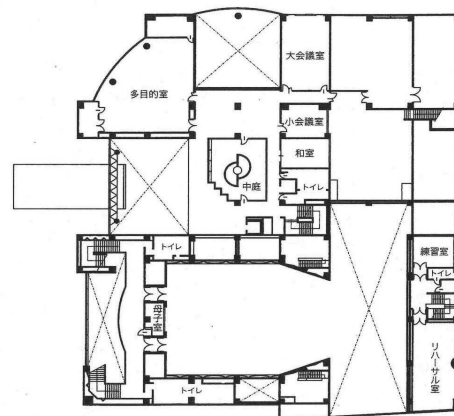
2階平面図
