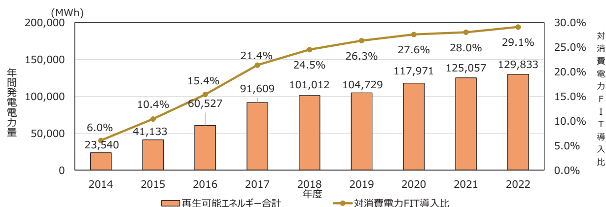
■再生可能エネルギーの年間発電量と対消費電力FIT導入比の推移
